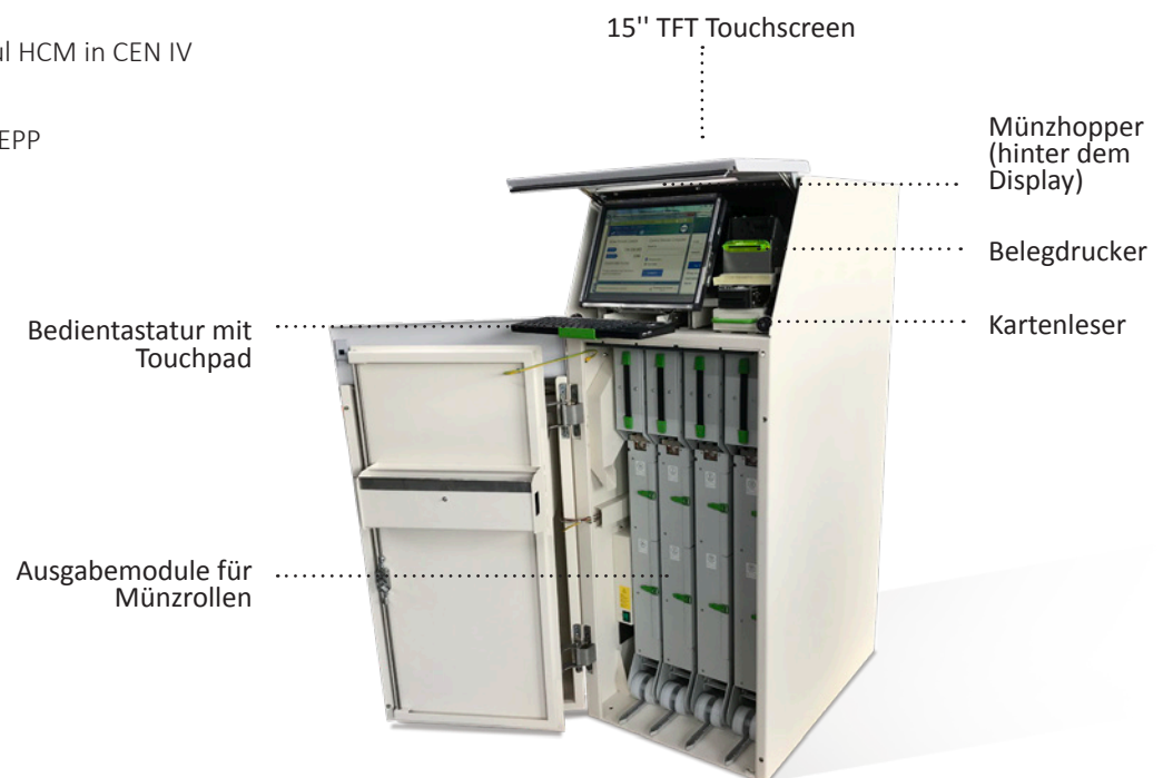
Version CRC-2610 Frontzugriff mit Ausgabe von Münzrollen
